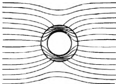
Permeabiliteit.
